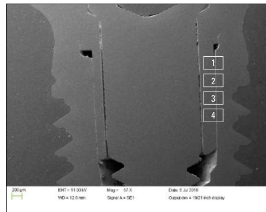
Fig. 2 Immagine al SEM con aree di riferimento contrassegnate nella sezione B (potere di ingrandimento 57x): impianto-abutment compatibile. I quadrati evidenziano le 4 aree prese in esame, che verranno indicate nel corso dello studio come area 1, 2, 3 e 4.
